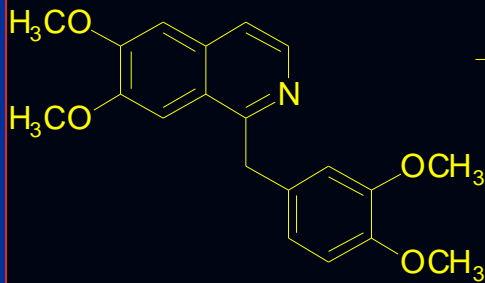
PAPAVERINA
