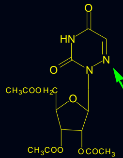
AZARIBINA
