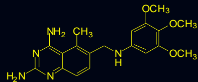
TRIMETRE XATO
