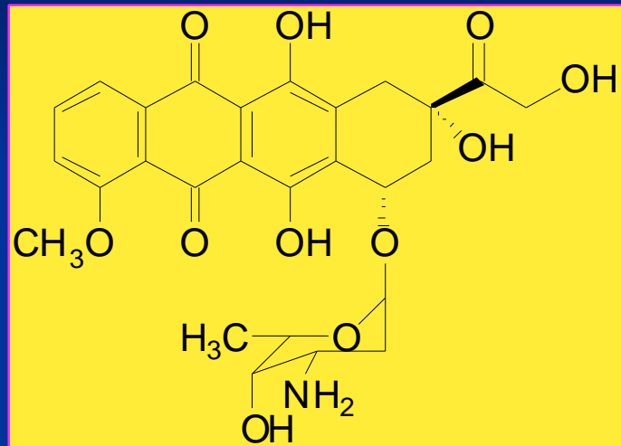
DOXORUBICINA
