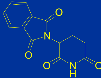
TALIDOMIDA (antiangiogénico)
