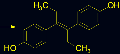
ESTILBESTROL
