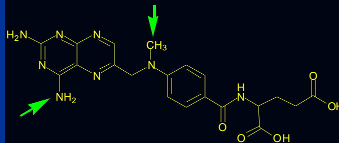
METOTREXATO
