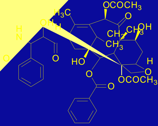
TAXOL
