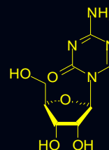
5-AZACITIDINA
