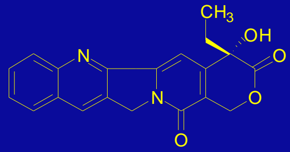
CAMPTOTECINA
