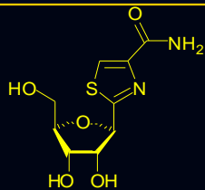
TAZOFURINA
